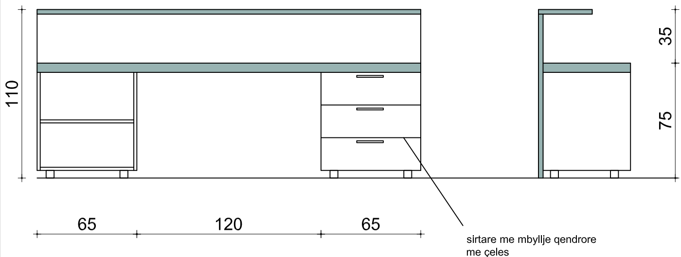
prerje 1-1
